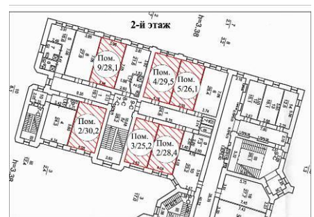
Схема местоположения помещений с печами на ПИБ 2005 г., 2 этаж
