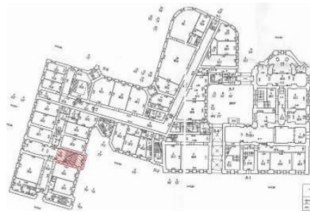
Местоположение Лестницы Л4 на ПИБ 2005 г., 1 этаж
