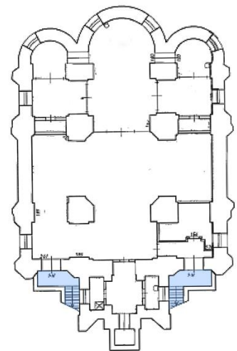
План подвала
