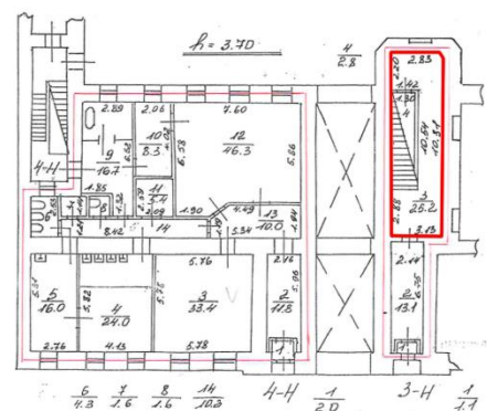
План 1 этажа
