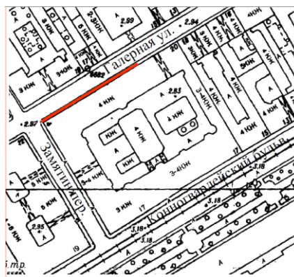
Ситуационная схема
