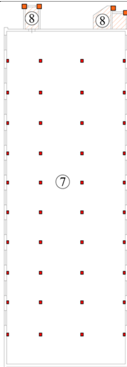
План надсилосного этажа
