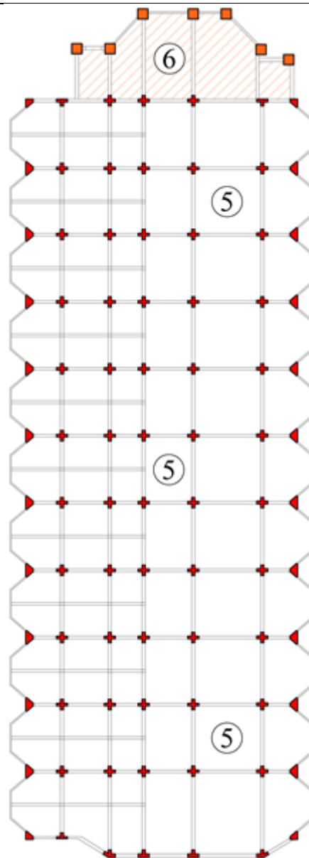
План силосного этажа
