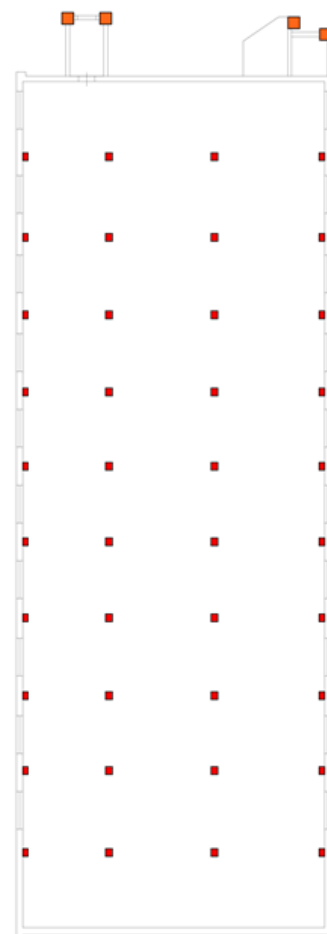
План надсилосного этажа
