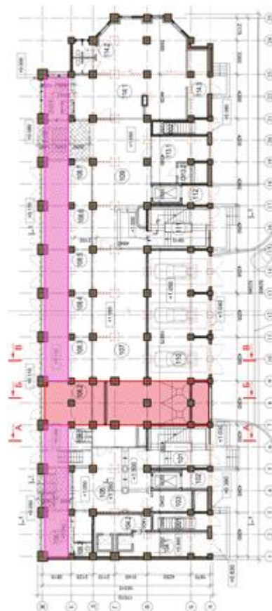
План подсилосного (первого) этажа
