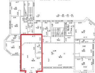
План 1 этажа
