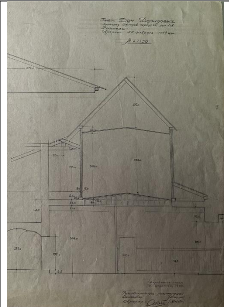
Фрагмент обмеров 1948 г.
