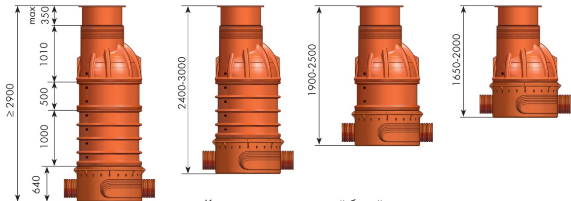
Колодцы с плосдонной базой
