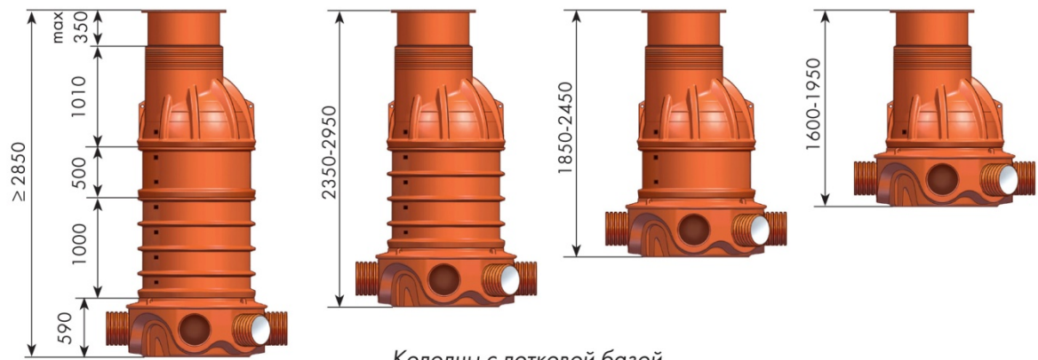
Колодцы с лотковой базой
