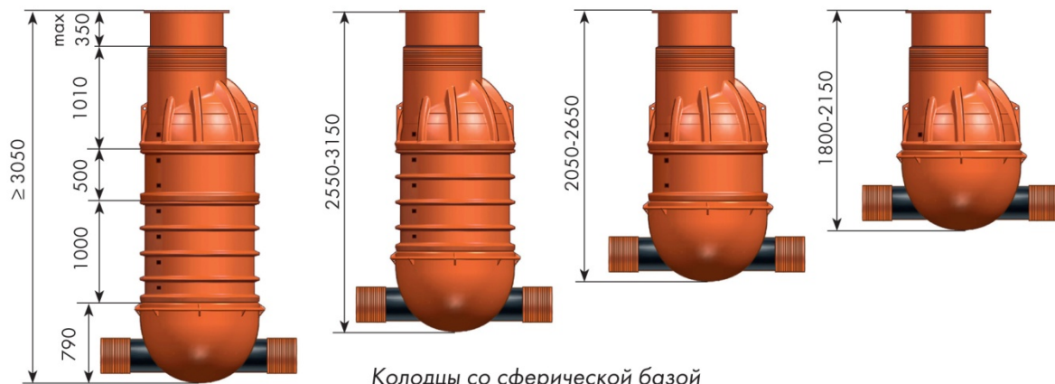
Колодцы со сферической базой
