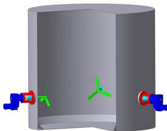
Боковые перемешивающие устройства
