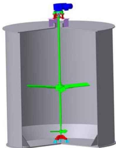
Вертикальные перемешивающие устройства
